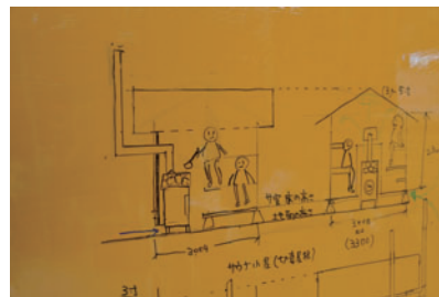
3×3mのハンドカットログをサウナ小屋として使うためのイメージ図。ロググラフはサウナづくりも得意なメーカーだ
